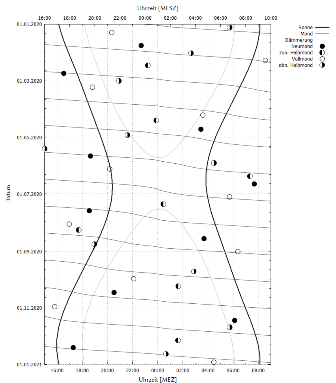
Untergänge
