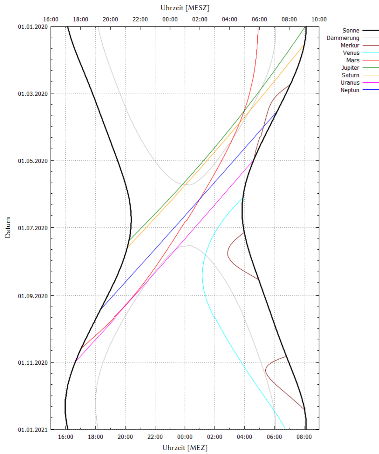
Aufgänge
