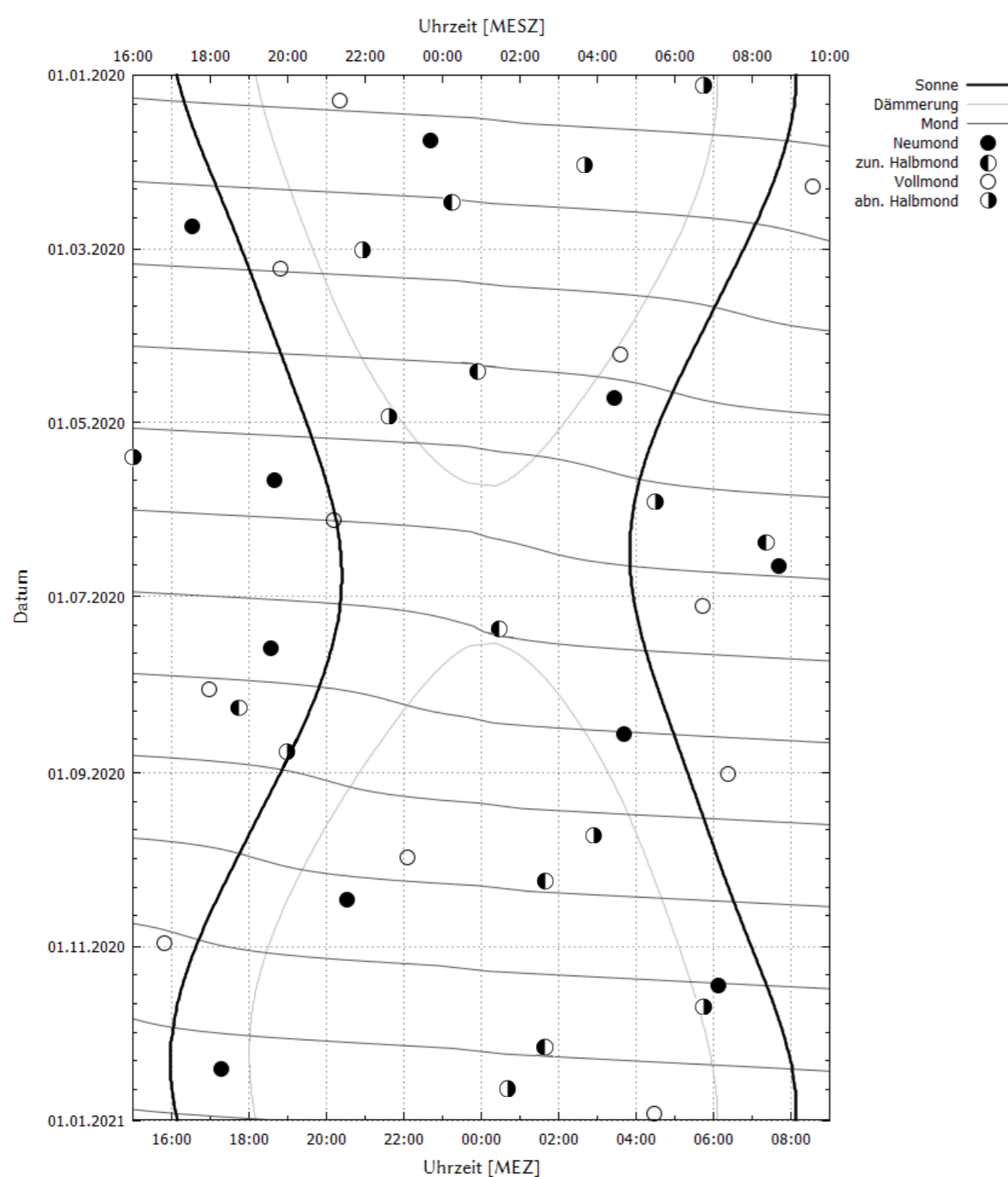
Aufgänge
