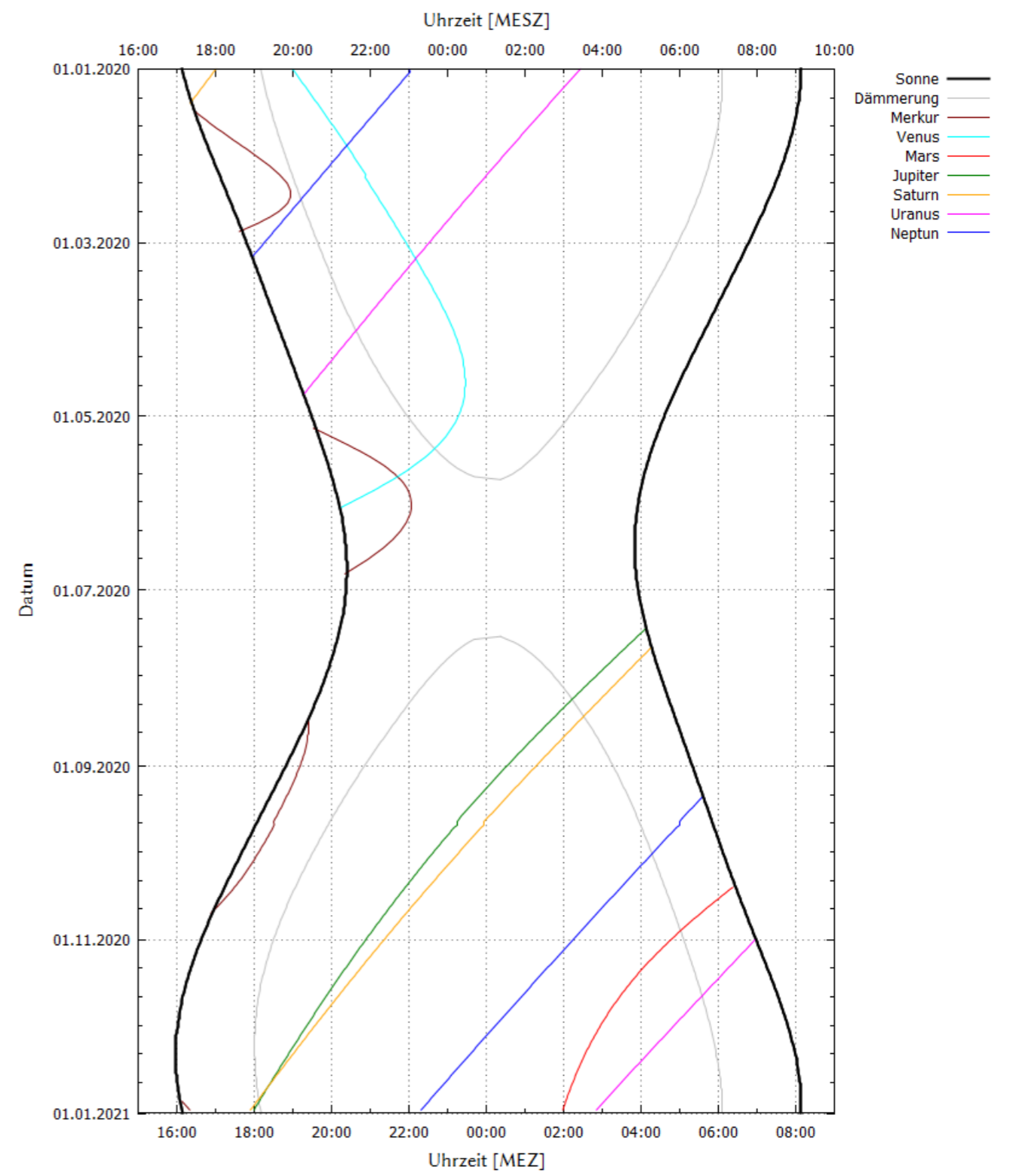
Untergänge
